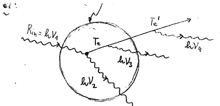
Slika 30: Energijska bilanca kerme v volumnu V . Vpadni foton R_{in} = h\nu_1 interagira v volumnu; nastali nabiti delci (npr. elektron s kinetično energijo T_e ) in sipani/sekundarni fotoni ( h\nu_2, h\nu_3, h\nu_4, T'_e ) zapustijo volumen.
