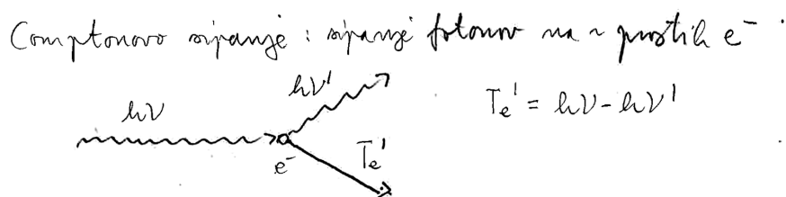
Slika 4: Skica Comptonovega sipanja. Vpadni foton h\nu se siplje na elektronu v smer h\nu' in mu preda del svoje energije; kinetična energija Comptonovega elektrona je T_e' = h\nu - h\nu' .
