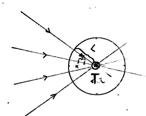
Slika 24: Idealizirana postavitev z majhno detektorsko kroglico s presekom S okoli točke T . Vsak žarek, ki leti proti detektorju, prepotuje skozi absorbent pot dolžine L .
