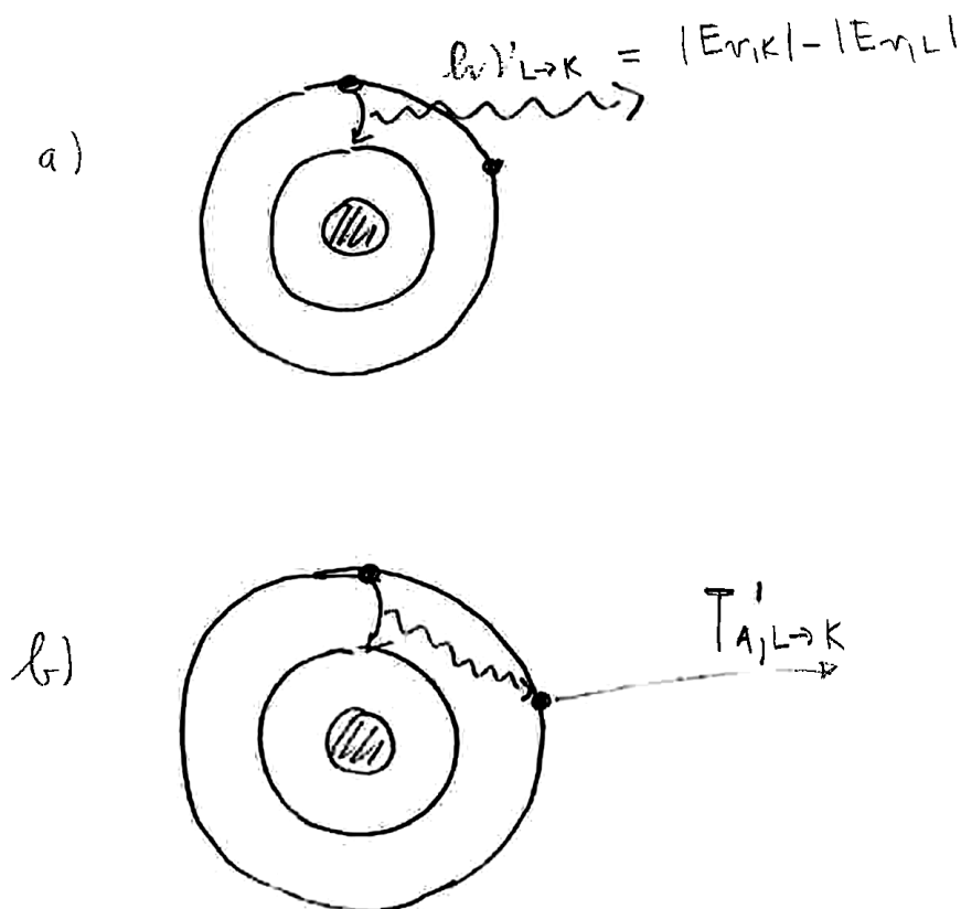
Slika 3: Relaksacija atoma z vrzeljo v lupini K. (a) Vrzal se zapolni z elektronom iz višje lupine L, razlika energij pa se izseva kot karakteristični žarek X z energijo h\nu'_{L\rightarrow K} = |E_{v,K}| - |E_{v,L}| . (b) Energija se prenese na elektron v višji lupini, ki ga izbije kot Augerjev elektron s kinetično energijo T'_{A,L\rightarrow K} .
