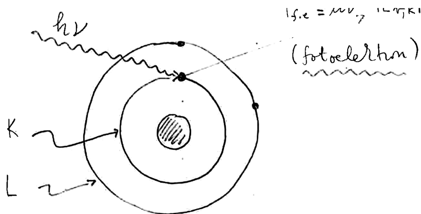
Slika 2: Fotoelektrični pojav. Vpadni foton h\nu izbije elektron iz notranje lupine (K ali L), pri čemer v atomu ostane prazno mesto (vrzel). Kinetična energija fotoelektrona je T_{f,e} = h\nu - |E_{v,K}| .
