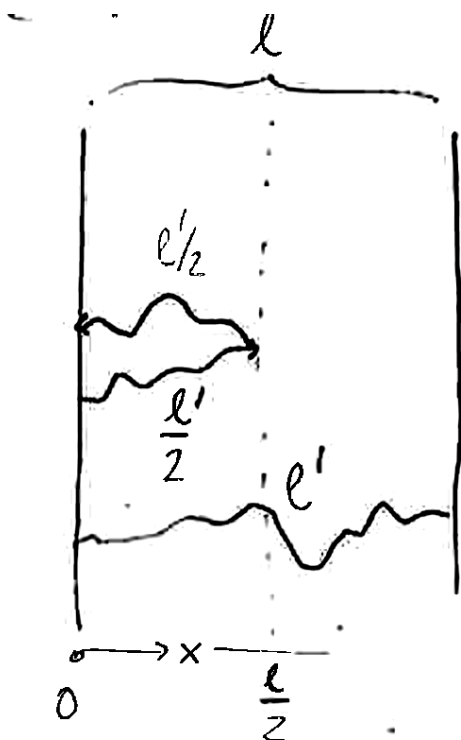
Slika 42: Vpliv povratnega sipanja v tanki plasti. Elektron se v povprečju povratno siplje na globini x \approx l/2 ; skupna prepotovana dolžina v plasti ostane l'/2 + l'/2 = l' .
