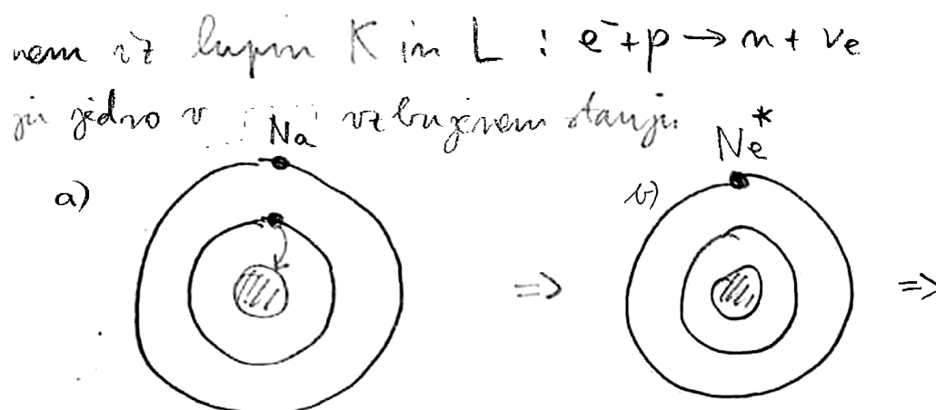
Slika 7: Zajetje elektrona (EC). (a) Jedro zajame elektron iz notranje lupine (najpogosteje K ali L) in odda nevtrino; nastane vzbujeno hčerinsko jedro. (b) Vzbujeno jedro {}^{22}\text{Ne}^* se relaksira z izsevanjem žarka gama.
